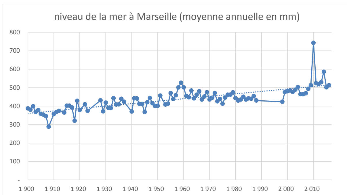
Figure 22 : élévation du niveau de la mer mesurée au marégraphe de Marseille
