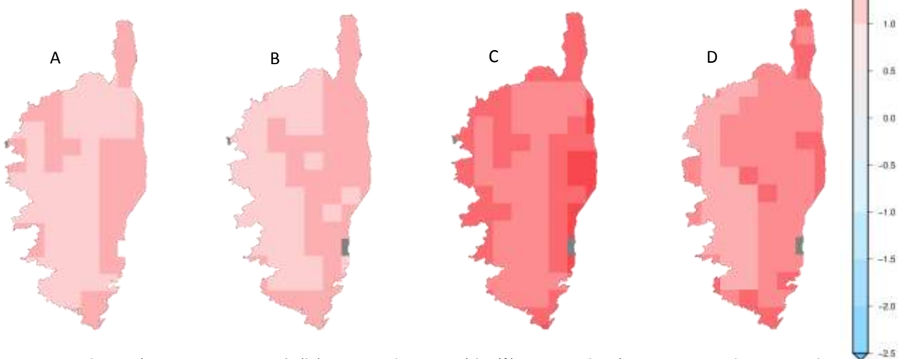
Figure 6 : Ecart de température moyenne estivale (°C) en Corse relativement à la référence, pour le scénario RCP4.5, aux horizons proches 2021-2050 avec le modèle Aladin (A) ou WRF (B) et aux horizons lointains 2071-2100 avec le modèle Aladin (C) ou WRF (D). Extraits de la plateforme DRIAS.
