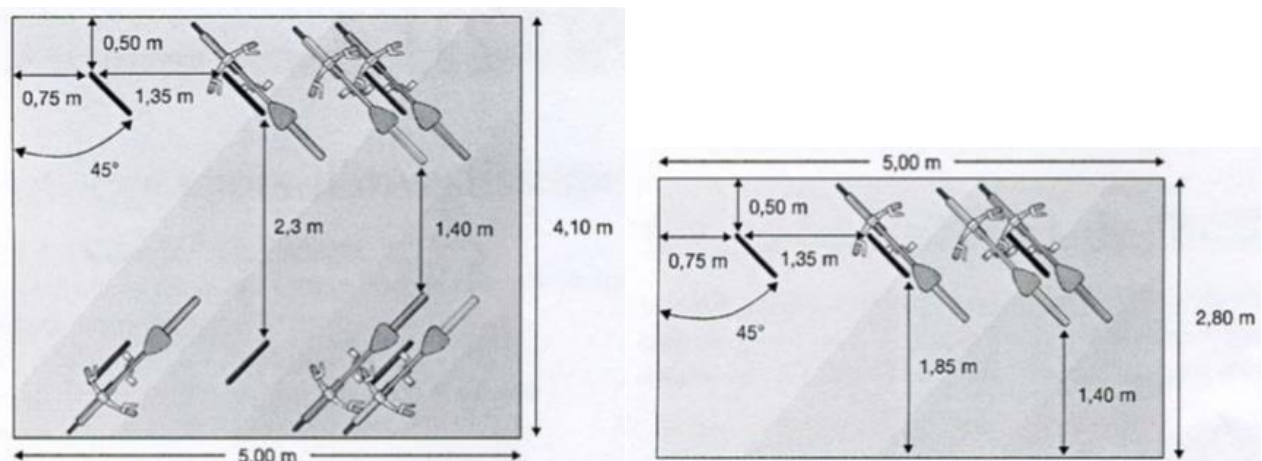
Dimensionnement type d'un parking pour deux-roues (source : CERTU "interface urbanisme et déplacements")
