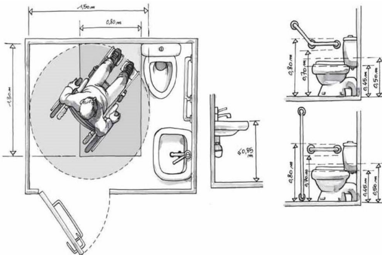
Principe d'aménagement d'un sanitaire PMR
