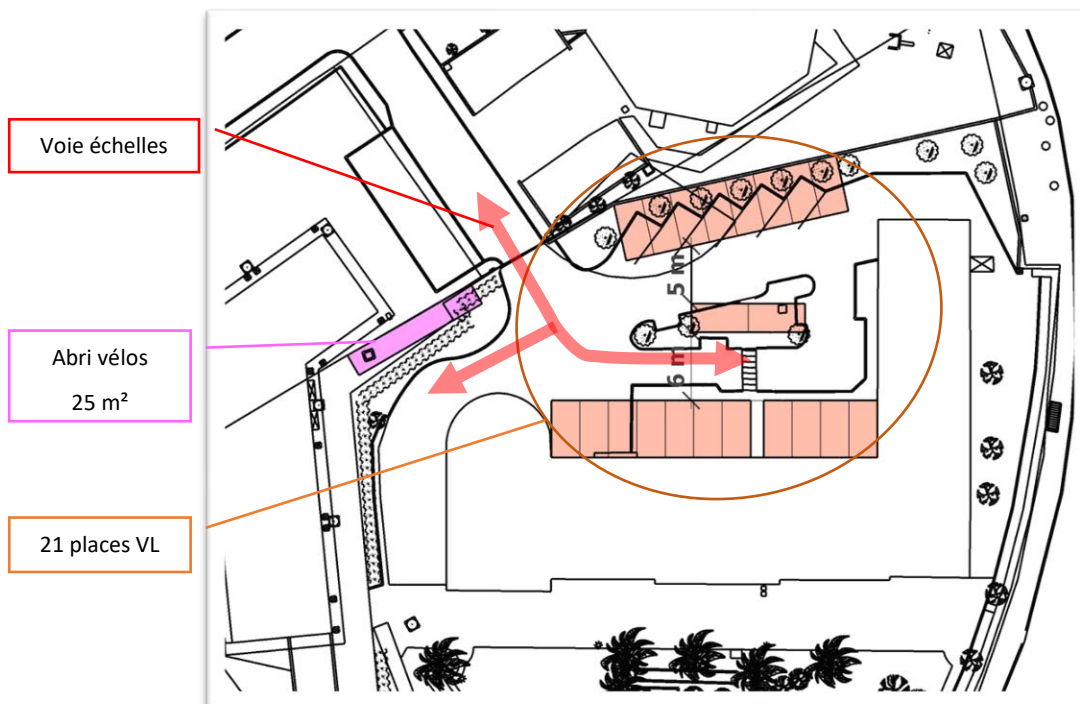
Illustration 42 : Principe d'implantation des stationnements sur site
