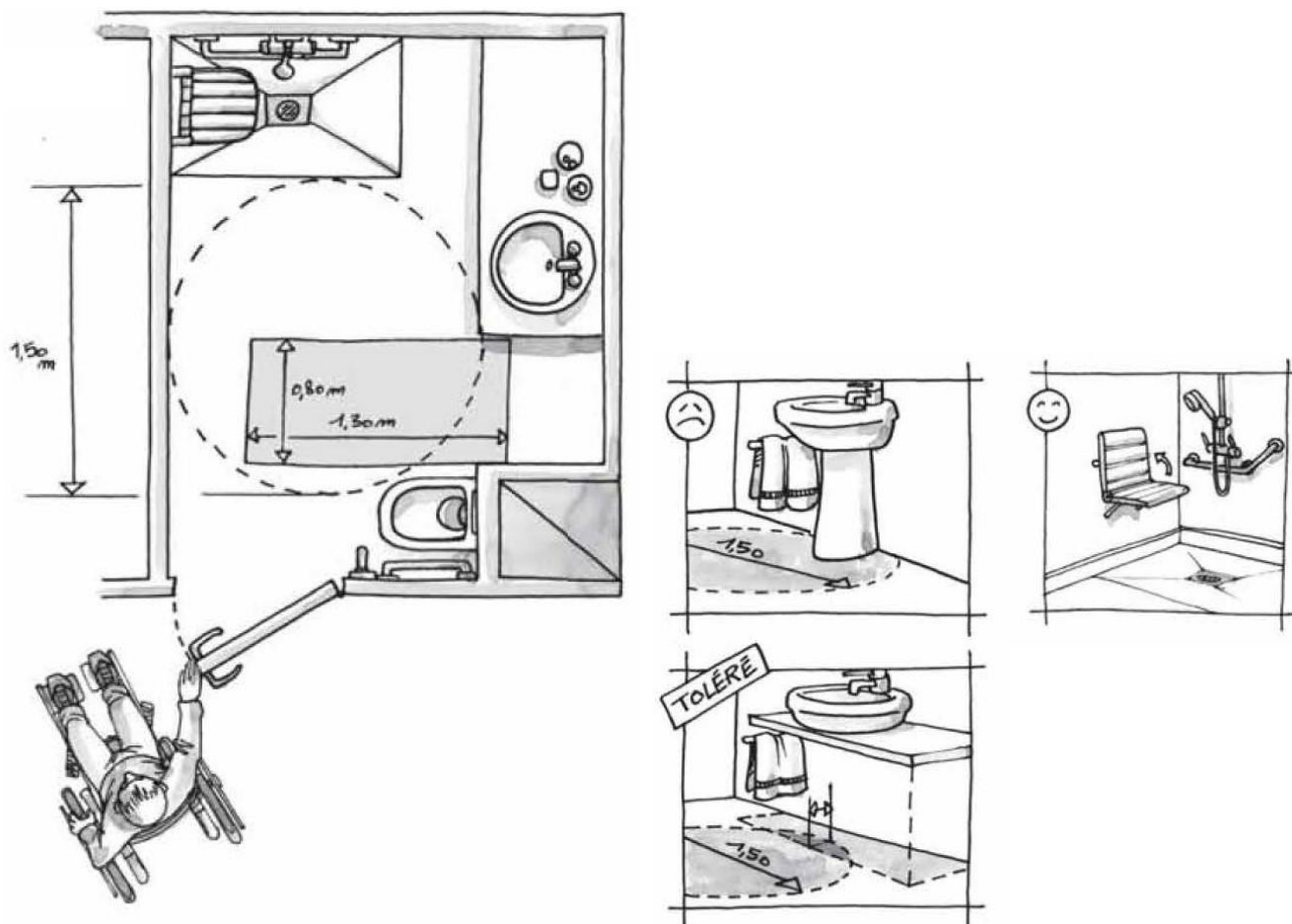
Schéma d'aménagement d'une salle d'eau accessible
