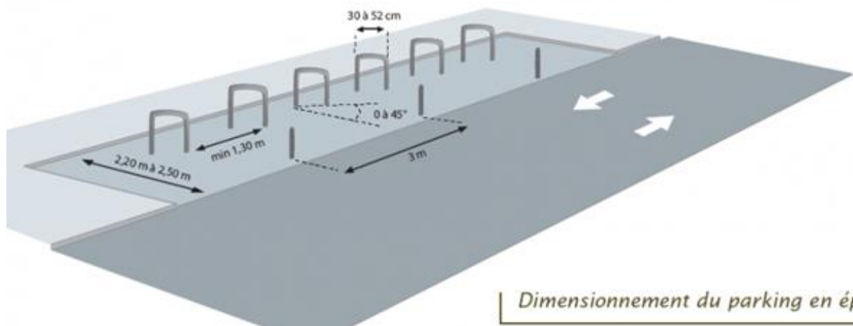
Dimensionnement type d'emplacements deux-roues (source : Institut Belge pour la Sécurité Routière)
