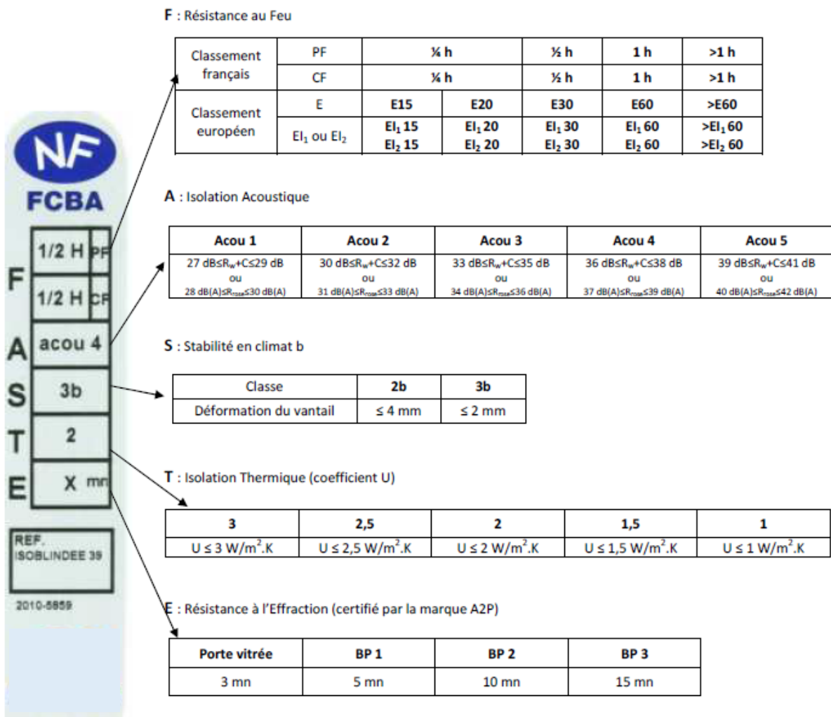
Principe d'étiquetage des portes – Classement FASTE
