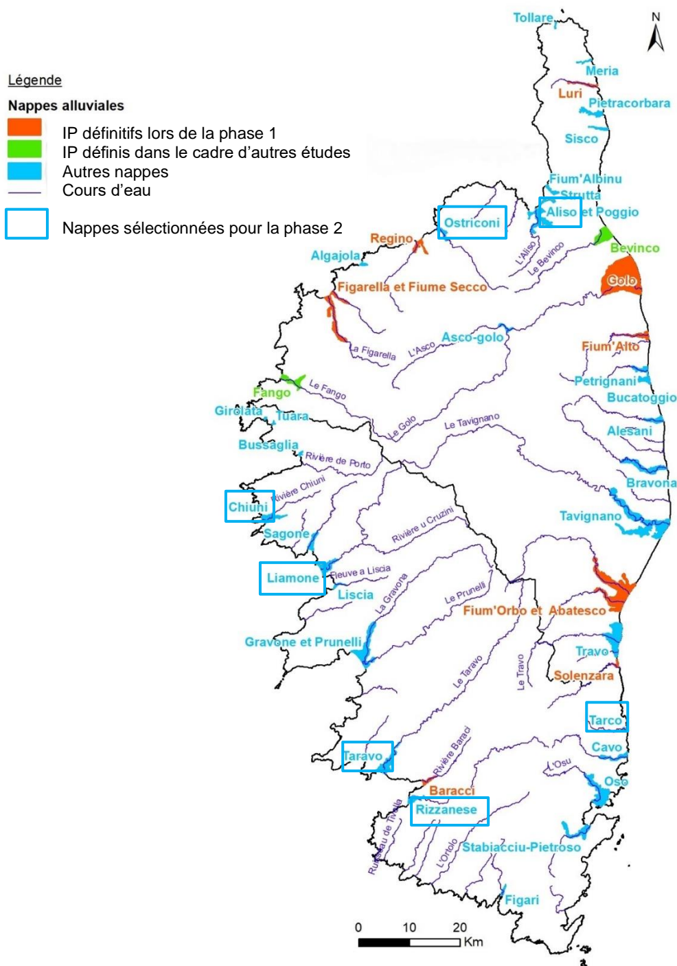
Illustration 1 : Nappes alluviales de la Corse
