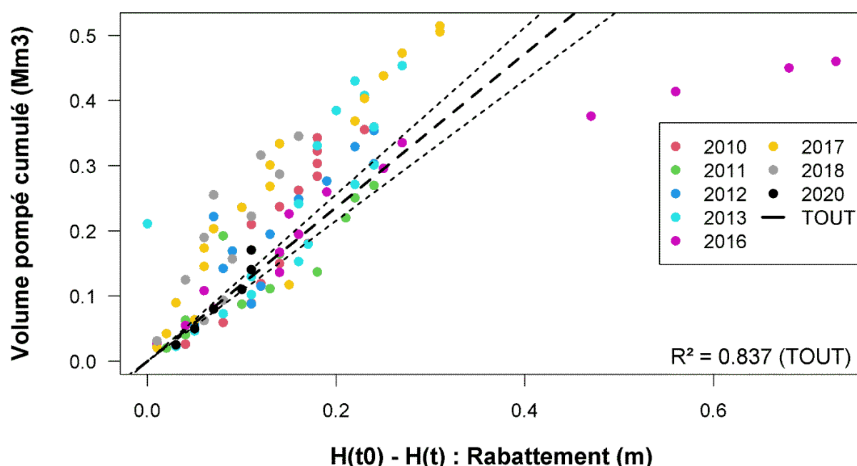
Illustration 3 : Evolution du volume pompé cumulé en fonction du rabattement pour la nappe alluviale du Fium'Alto
