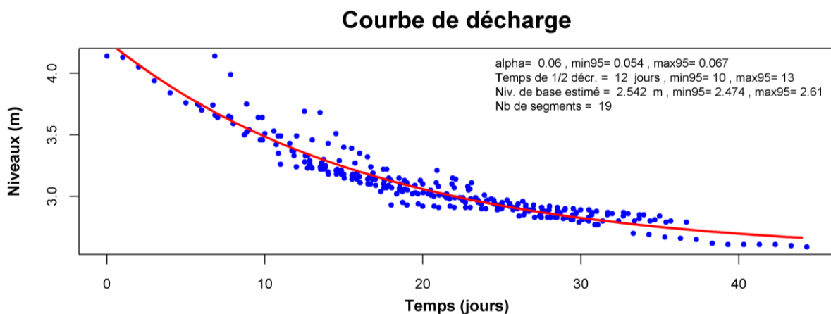
Illustration 2 : Courbe de décharge relative à la nappe alluviale du Fium'Alto
