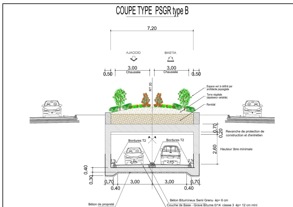
Solution retenue : PSGR type B bidirectionnel sens RT 21 / RT 40
