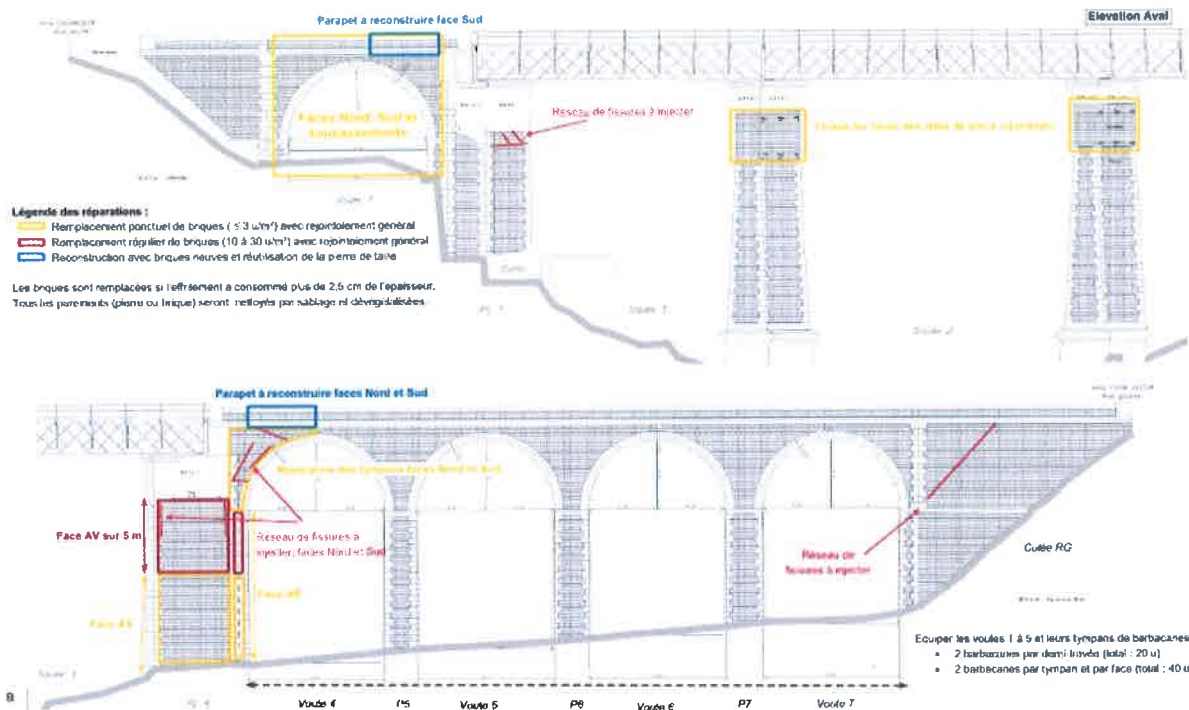
Exemple de travaux de maçonneries (Prunelli)
