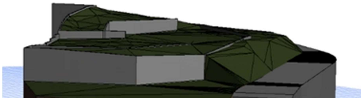
Modélisation du terrain, vue du Sud (murs de soutènement en premier plan + soutènement de la plateforme haute)
